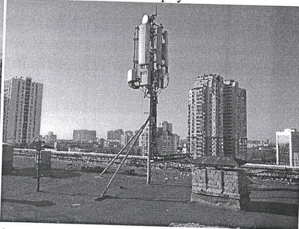
частина даху
